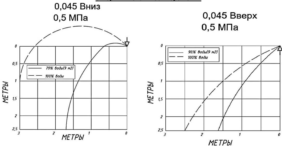
График зависимости интенсивности орошения от давления на площади 9 м2, защищаемой одним распылителем с высоты 2,5 м
